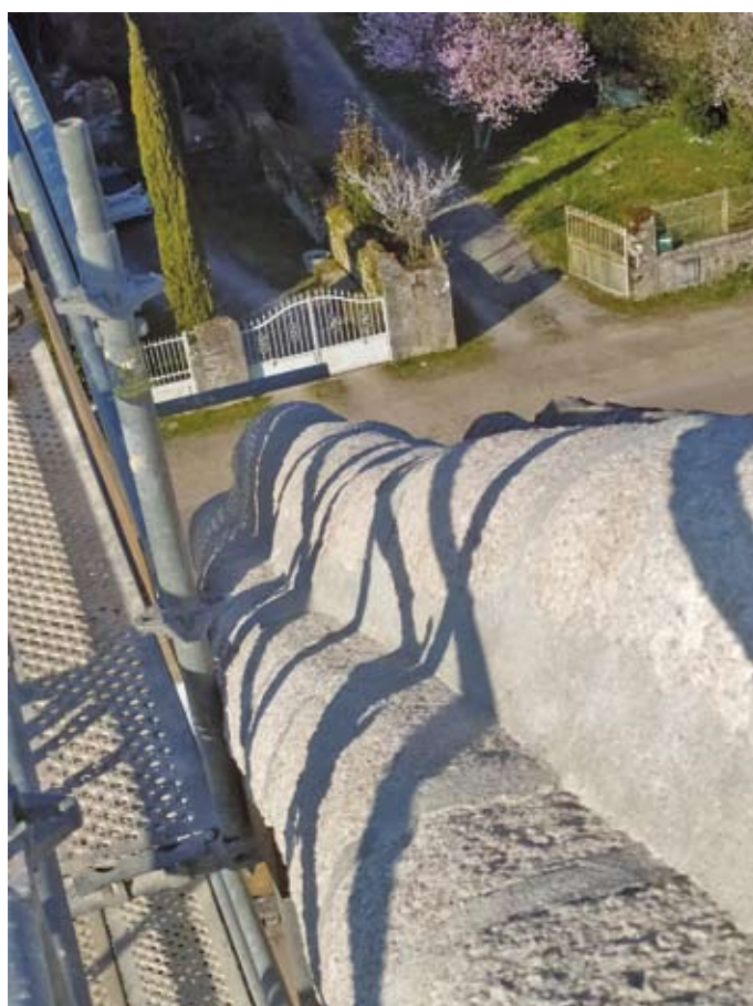
Démoussage et rejointement du fronton vus du haut des échafaudages (7 mars 2022)
